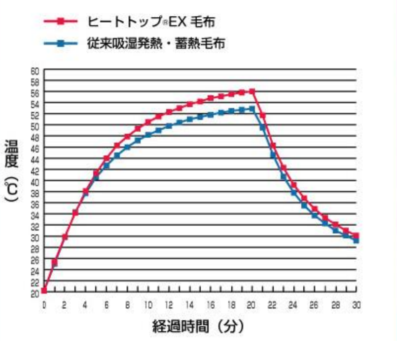
製品【ヒートトップ®EX】吸湿発熱性の比較データ
