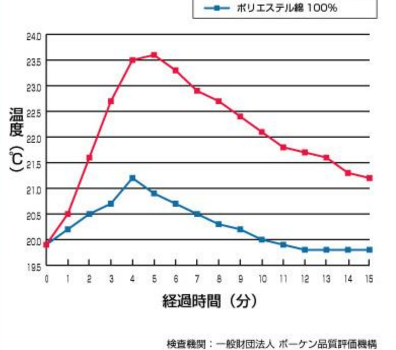
吸湿発熱わた【ヒートトップ®EX】吸湿発熱性の比較データ
